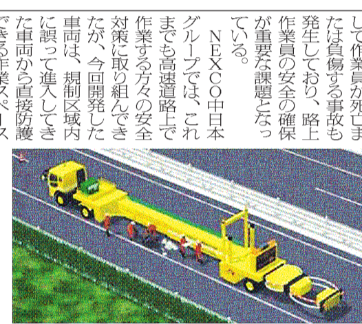
大型移動式防護車両 (左：走行時、右：作業時)
